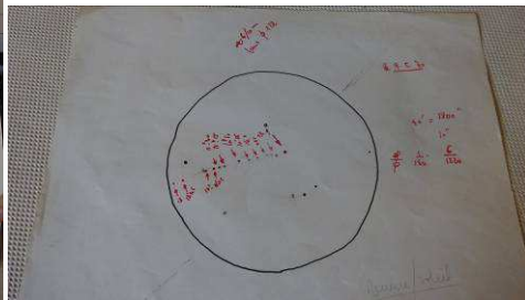
Dessin réalisé par Mr Noël Transit de mercure le 9 mai 1970 observé avec une petite lunette terrestre par projection
