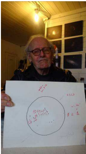
Dessin réalisé par Mr Noël Transit de mercure le 9 mai 1970 observé avec une petite lunette terrestre par projection
